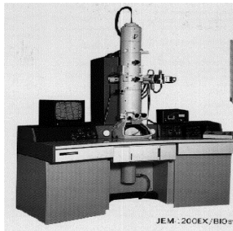
Fig. 6. Microscopio electrónico
