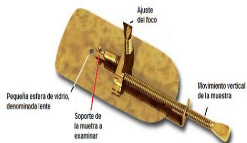
Fig. 2. Microscopio simple de Leeuwenhoek
