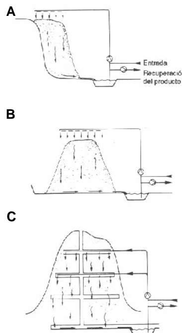
Fig. 2. Lixiviación mediante irrigación. A) Lixiviación en pendiente. B) Lixiviación en pilas. C) Lixiviación "in situ". Tomada de Crueger y Crueger, 1993.
